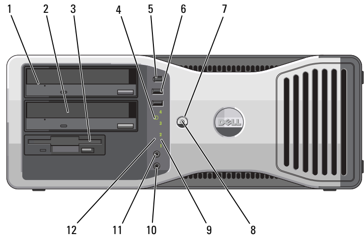
前視圖 ( 台式放置方式 )
